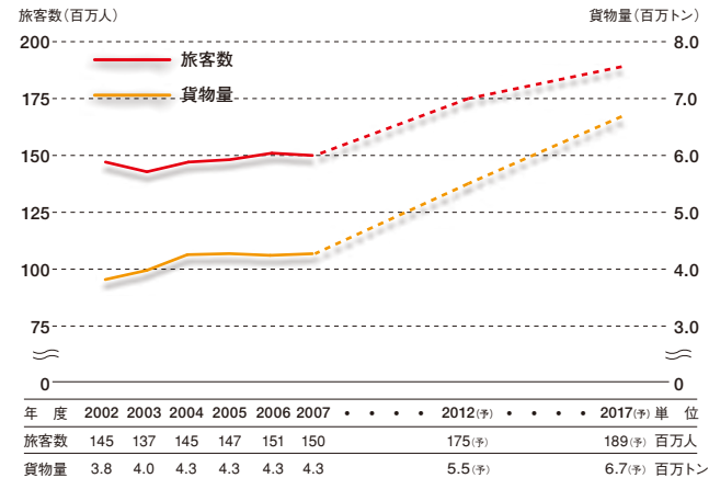
航空需要の推移と予測(旅客・貨物)
